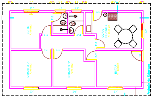
Figura 1 – Vista superior da casa. Fonte: Secretaria Municipal de Planejamento da Prefeitura de Goiânia, 2009.
