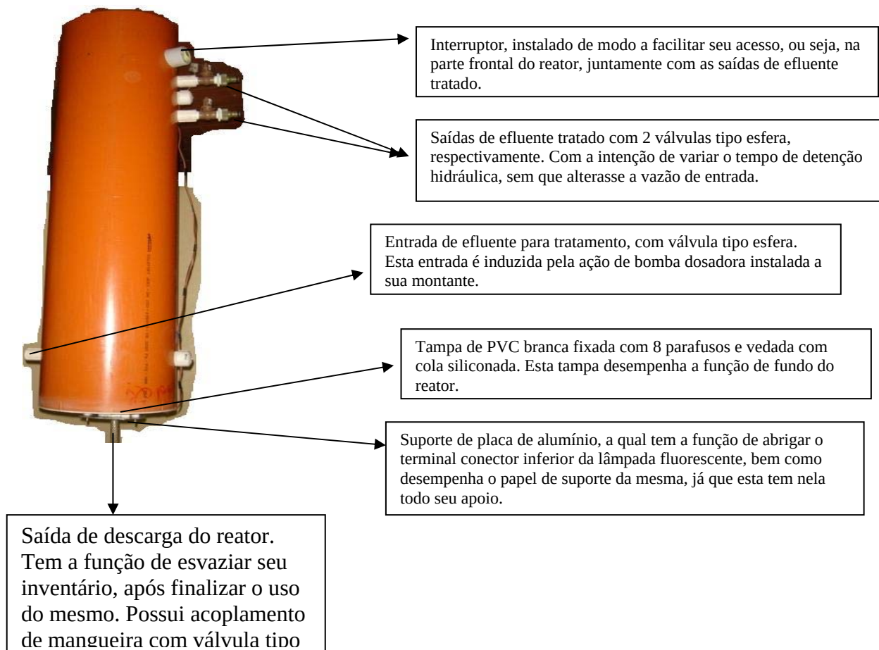
Figura 3: Explicação a respeito das partes componentes do reator fotocíclico.
