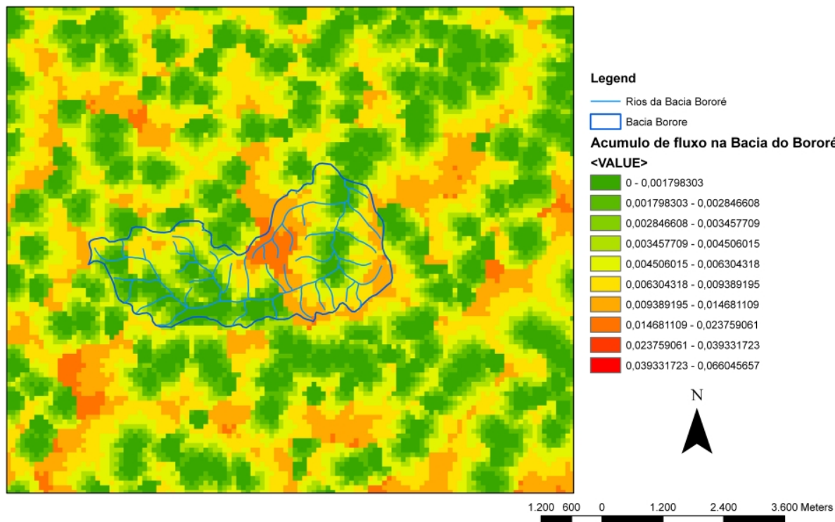
Imagem 1: acumulo de fluxos nos rios da bacia Bororé.
