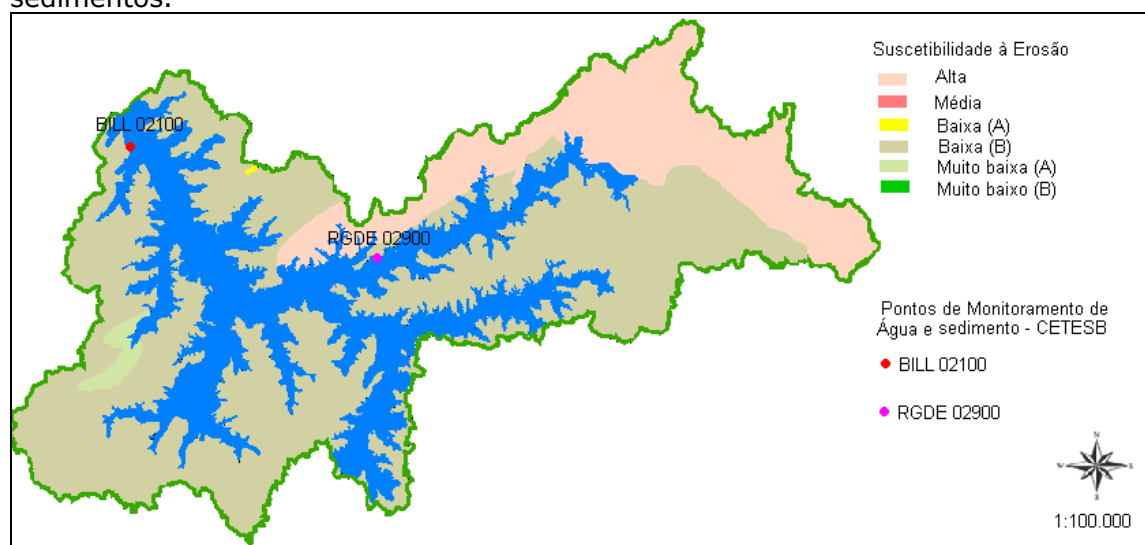
Figura 01: Suscetibilidade à erosão da Bacia Billings.(Elaboração própria).
