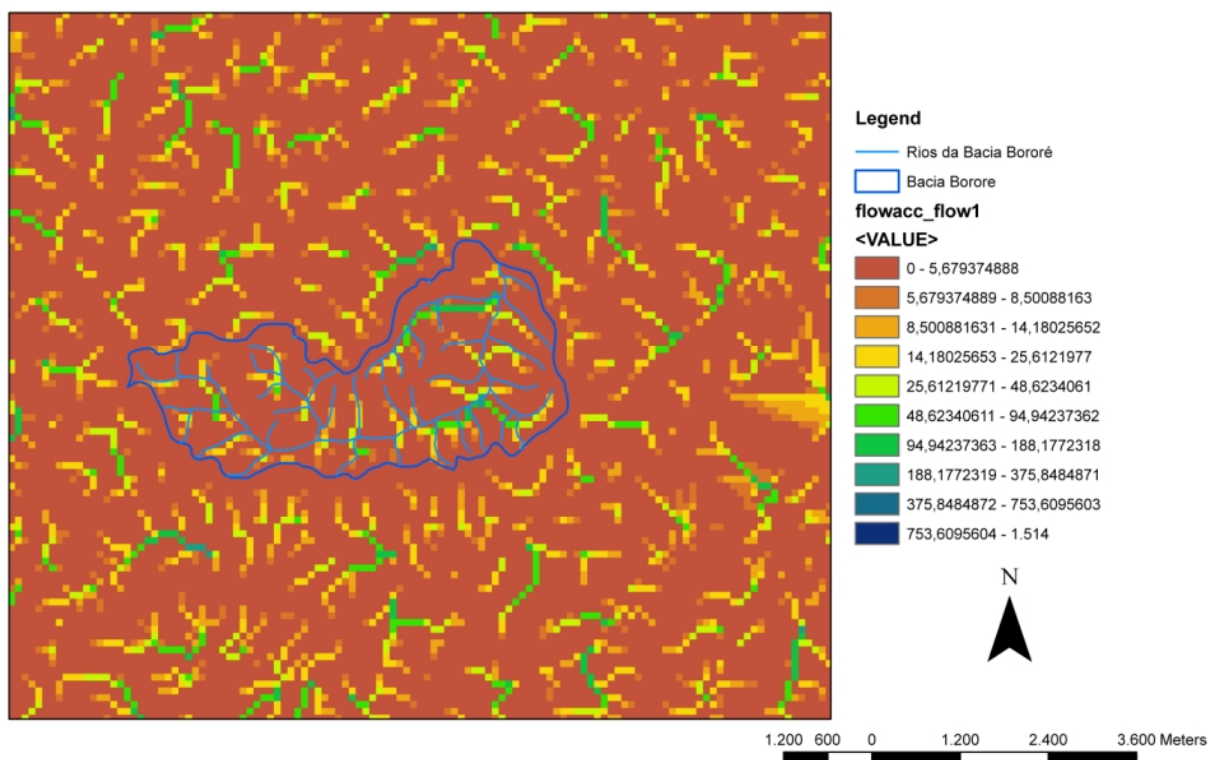
Imagem 2: tendencia de acúmulo de fluxo de sedimentos nos rios da bacia Bororé.
