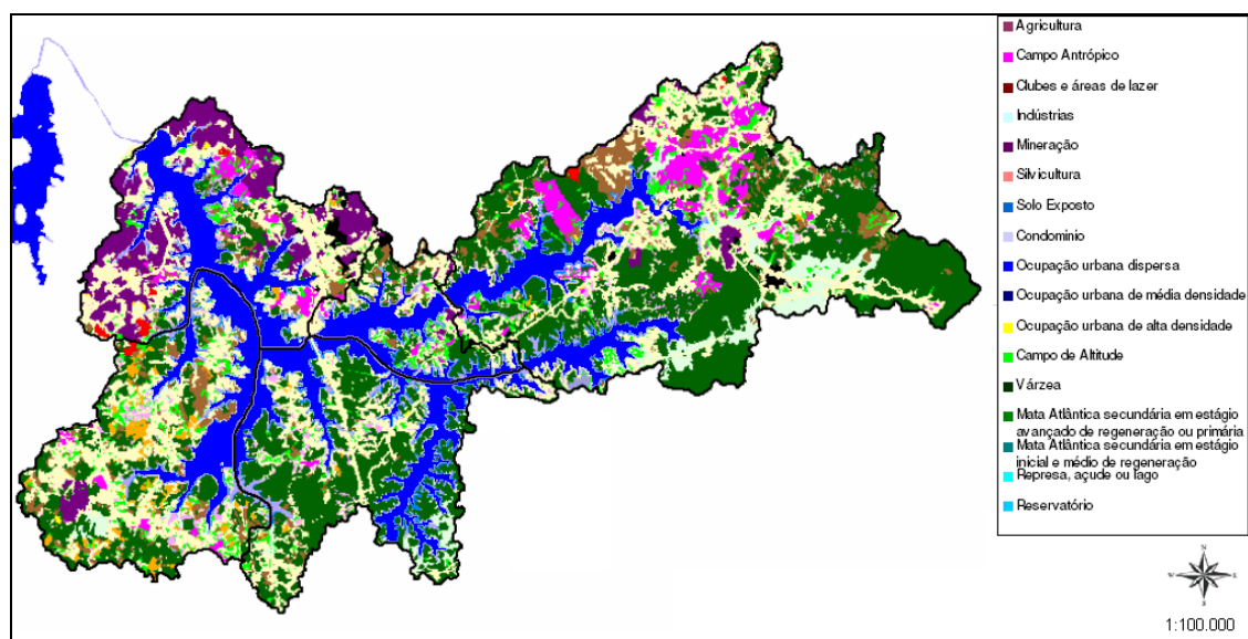
Figura 05: Uso e ocupação do solo na Bacia Billings (ISA, 2009).
