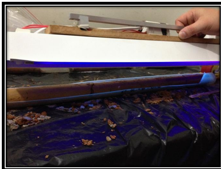
Figura 4. Lâmpada UV-A para detecção visual de produto na amostra de solo.
